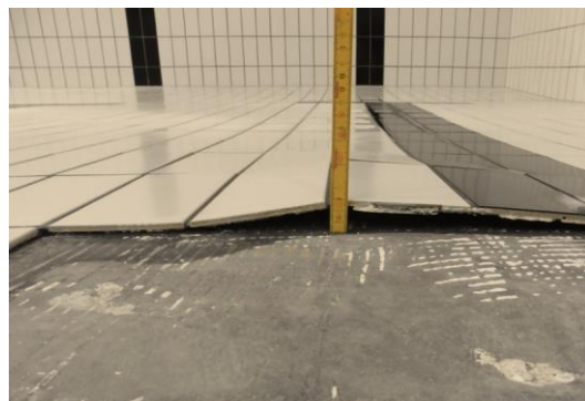
Figur 3: En betongkonstruksjon fortsetter å trekke seg sammen i flere år etter utstøping. (Illustrasjon: Sopro)
