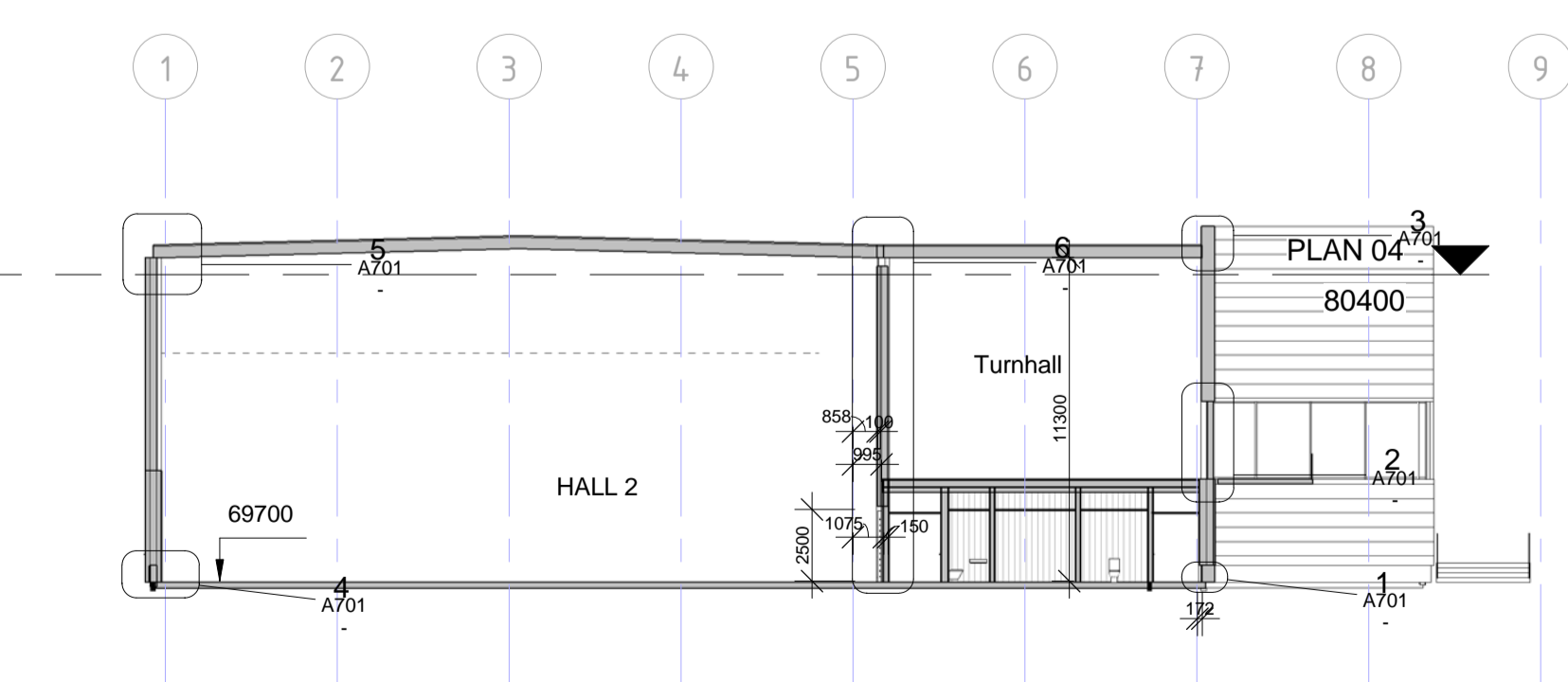
SNITT_E-E 1 : 250
