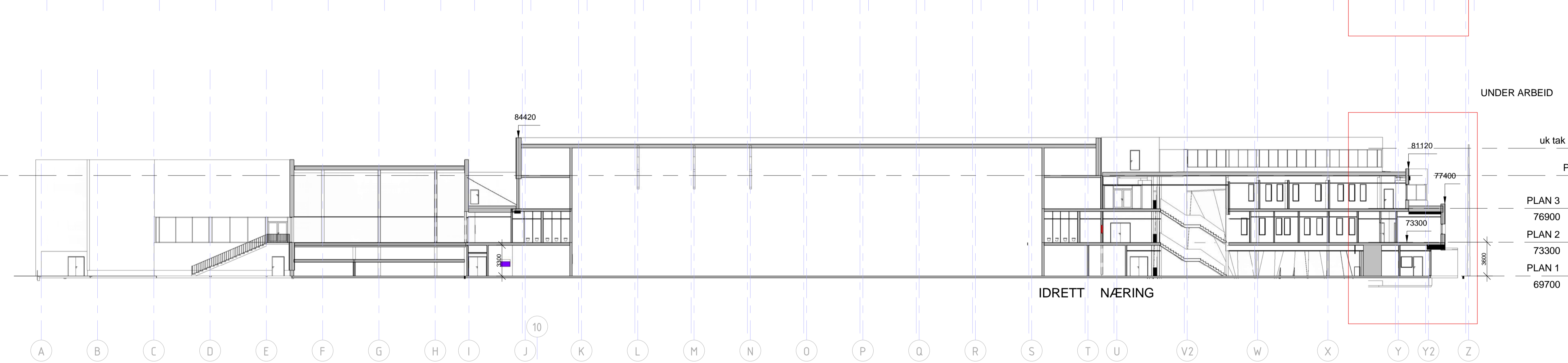
SNITT_8-8 1 : 250
