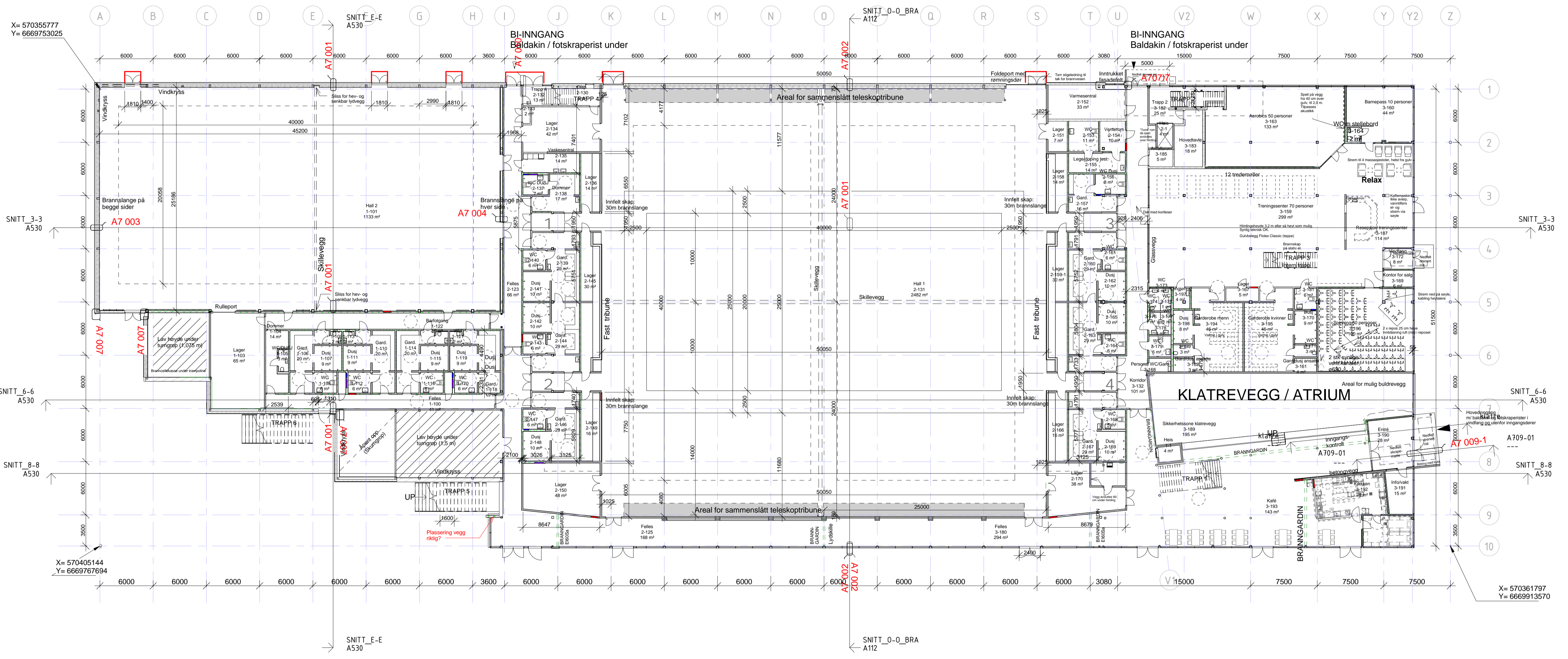
PLAN 01 1 : 250
