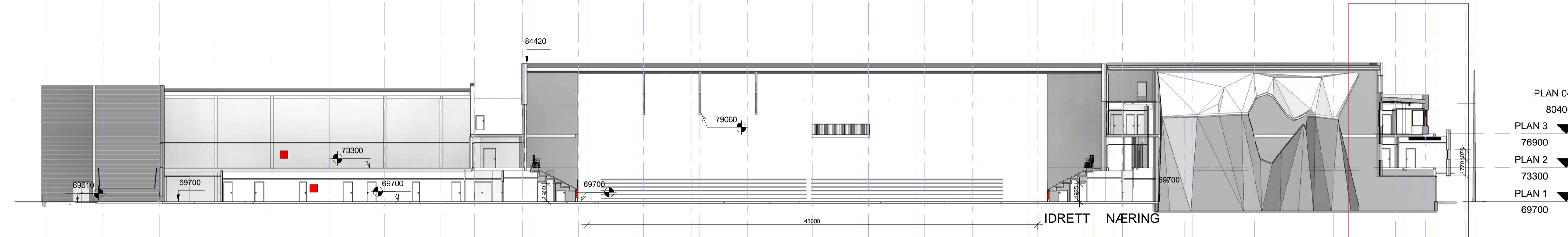
SNITT_3-3 1 : 250
