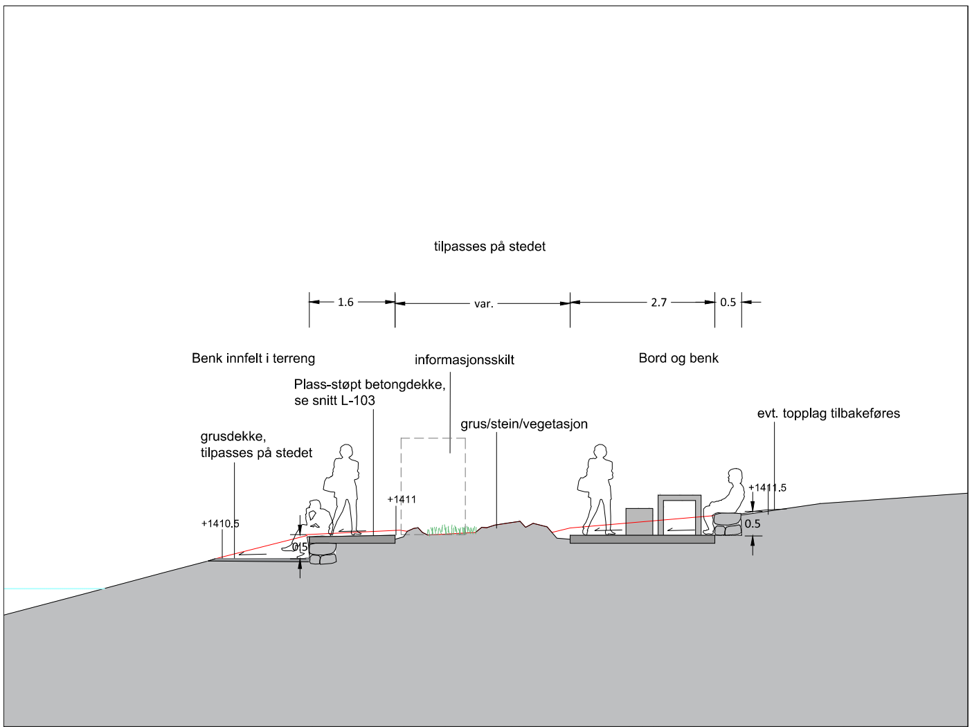
PRINSIPPSNITT E-E' Rasteplass nord
